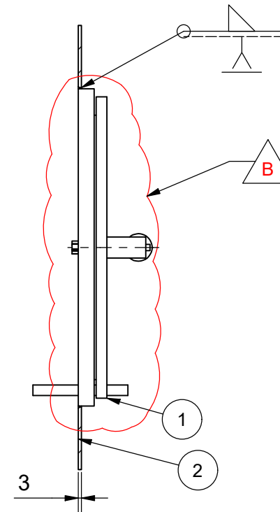
A-A ( 1 : 5 )
